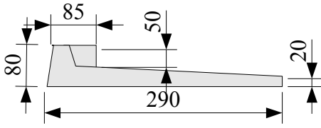
Seuil pour porte d'entrée
